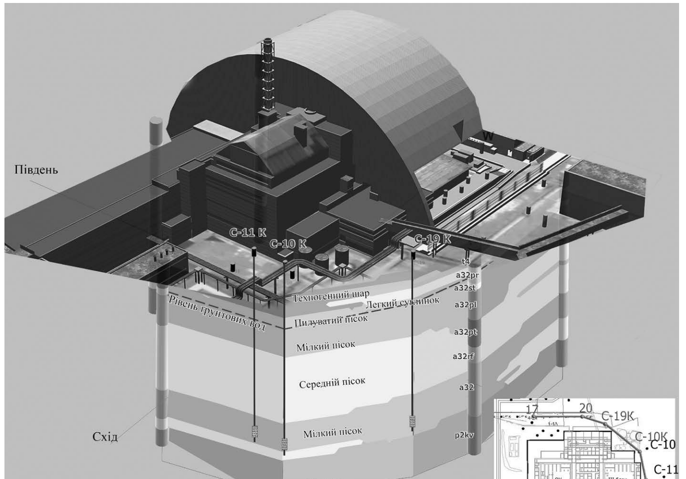
Рис. 4. Розташування нових куштів свердловин С-10к, С-11к, С-19к
